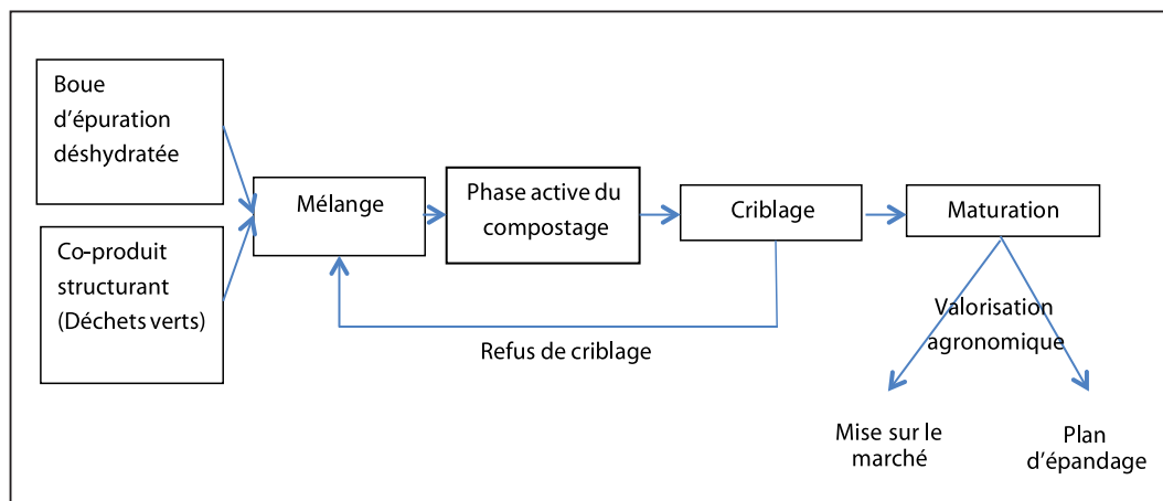
Schéma d'une filière de compostage type des boues d'épuration en France
