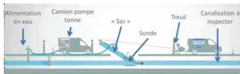
Inspection par champ lointain à l'aide de la sonde Inspect'O® (source : Aquadiag Solutions)
